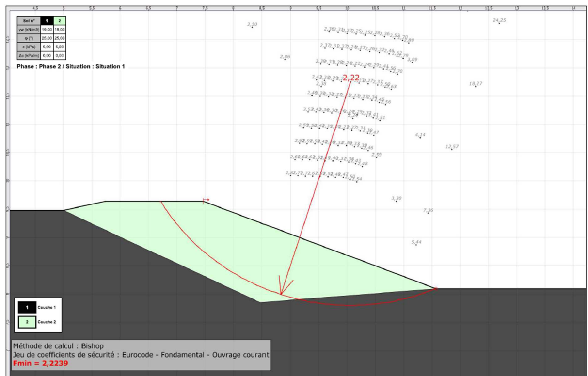
Résultat de calcul de stabilité (3H/1V) en phase définitive avec le logiciel TALREN
