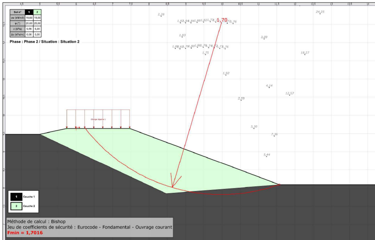
Résultat de calcul de stabilité (3H/1V) en phase provisoire avec le logiciel TALREN
